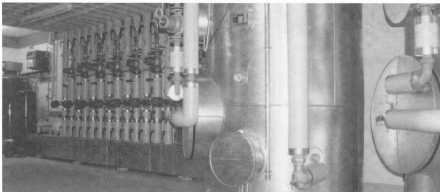
Heizungszentrale mit Warmwasseraufbereitung im Jugendhaus Seewis
