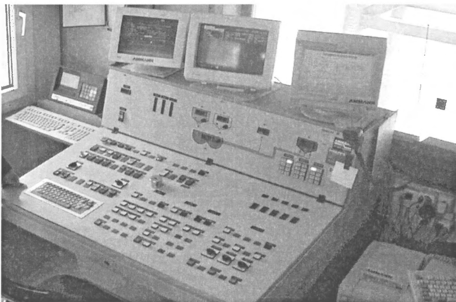
Hier haben die Computer das Sagen: Ausschnitt aus dem Kommandoraum mit dem Steuerpult für Dosier- und Betonanlage, Bildschirme für Dispo, Produktionssteuerung und Waage.
