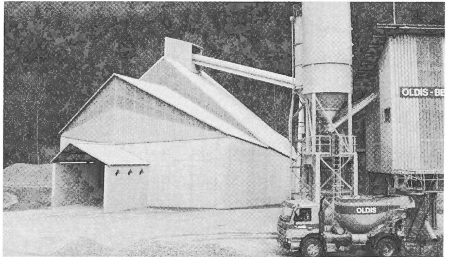
Ein Industriebau muss nicht hässlich sein: Brechsandsilo, Breite 26,5 m, Länge 32,5 m, Höhe 17,6 m, Nutzinhalt 3500 m 3 . Rechts: Betonanlage mit Zementsilos.
