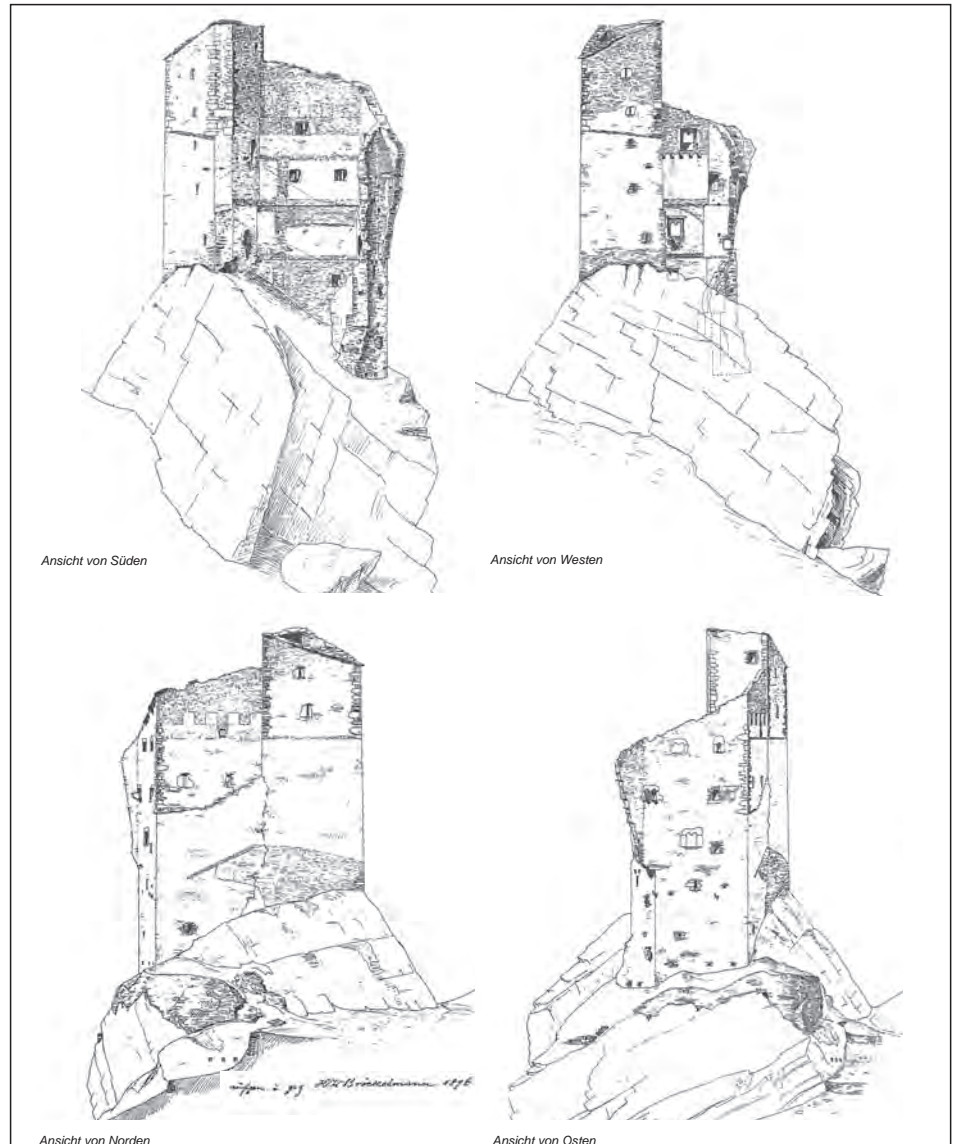
Abb. 6: Bauaufnahme dat. 1896 von H.W. Bröckelmann, Ansichten
