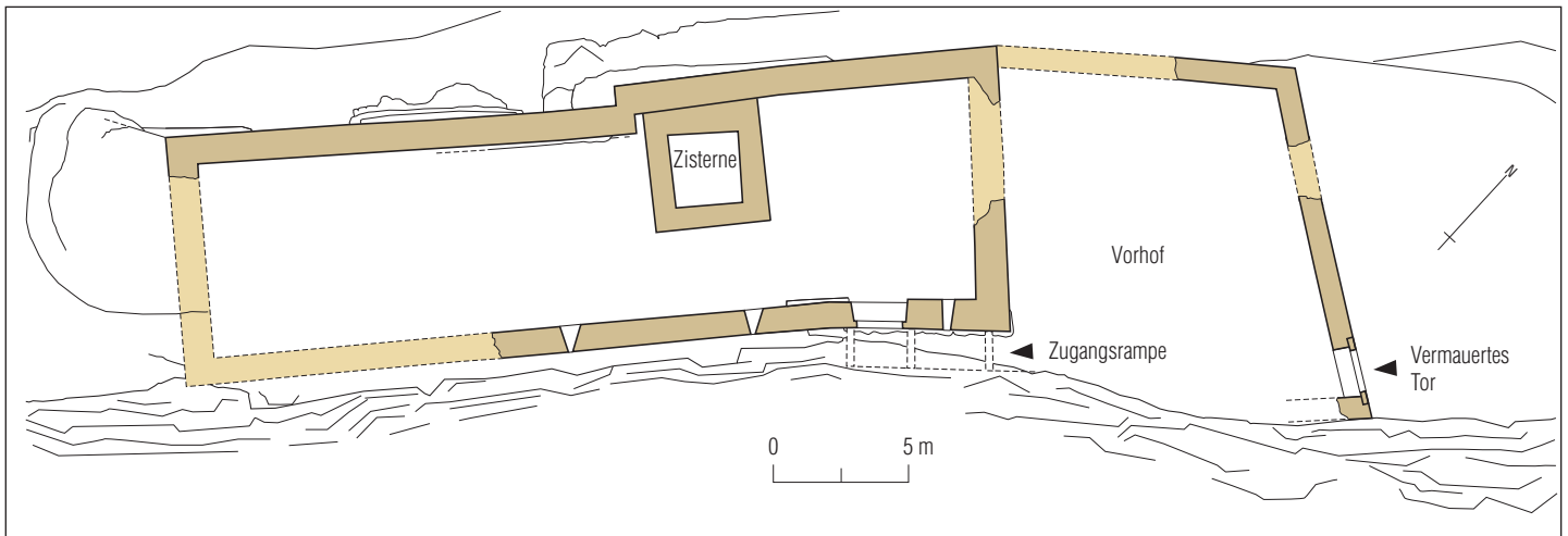
Abb. 18: Burg Lichtenstein, Grundriss Mst. 1:300 (Zeichnung Archäologischer Dienst GR)
